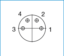
PIN分配
