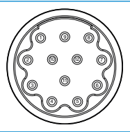
PIN分配
