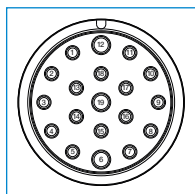
Occupazione PIN
