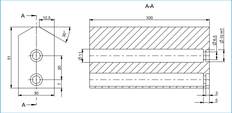
每个抓手钳口需要一个通用钳口
