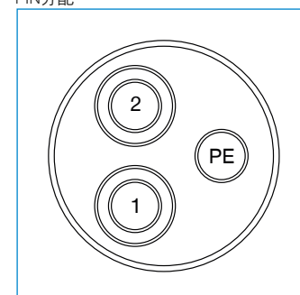
PIN分配
