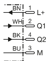
Schéma de raccordement
